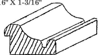
BB-11 11/16" X 1-3/16"
