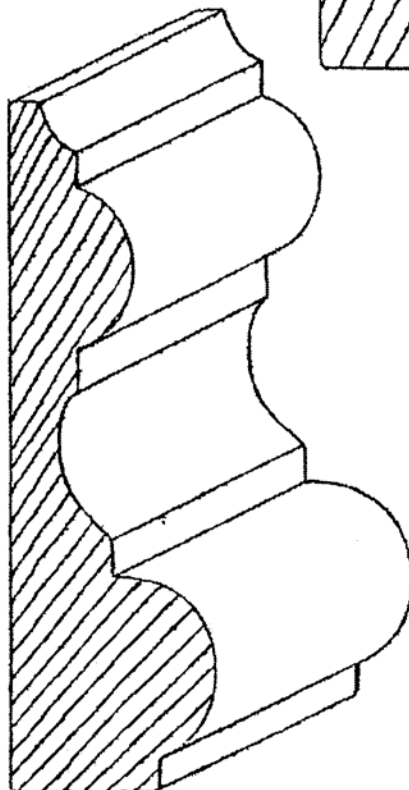
CAP-86 1-1/8" X 3-3/4"
