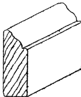
B-101 7/16" X 2"
