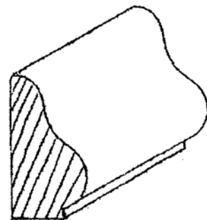
CAP-84 5/8" X 1-1/8"
